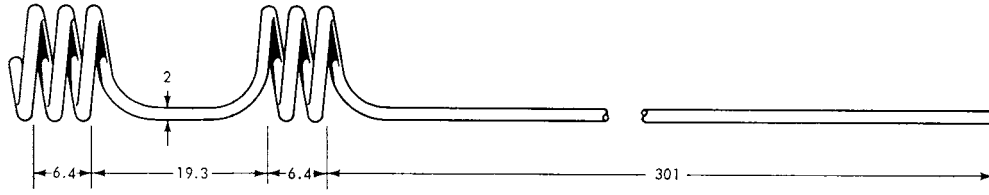
FIG. 2 Stirrer
