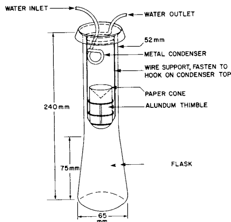
FIG. 1 Extraction Apparatus
