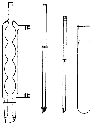
FIG. 2 Apparatus
