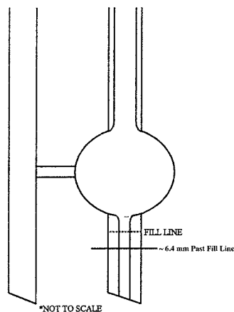
FIG. A3.1 Viscometer Fill Line
