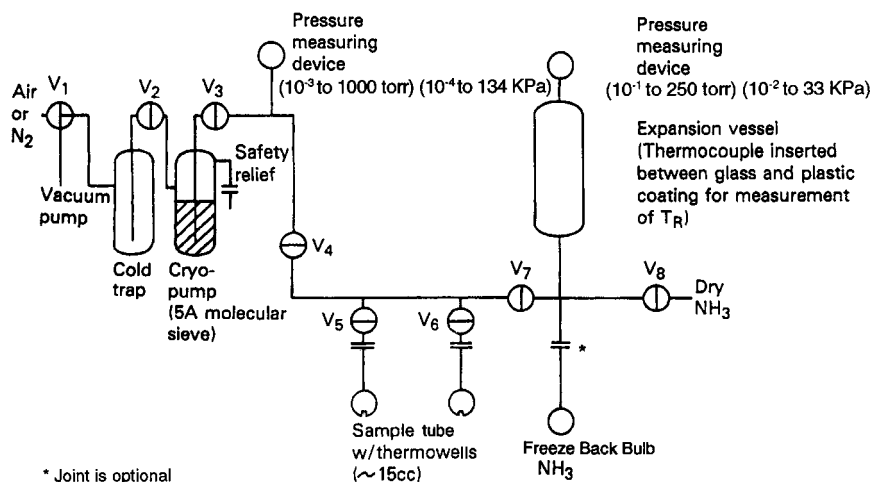
FIG. 1 Apparatus
